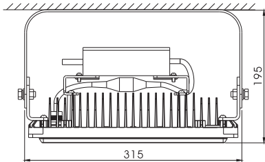
吸顶安装
